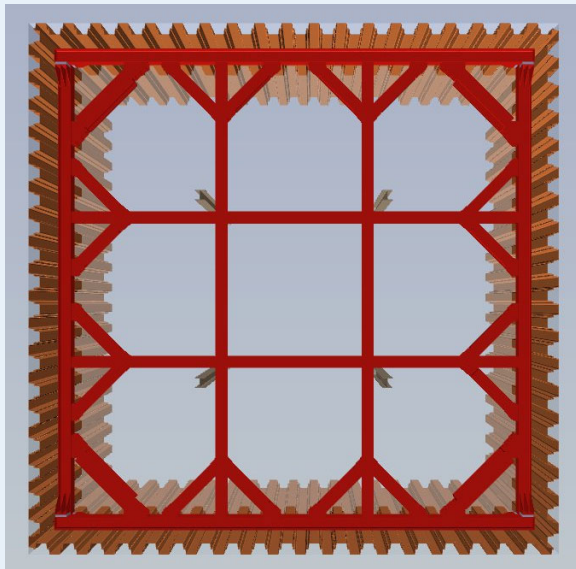
従来式山留材
